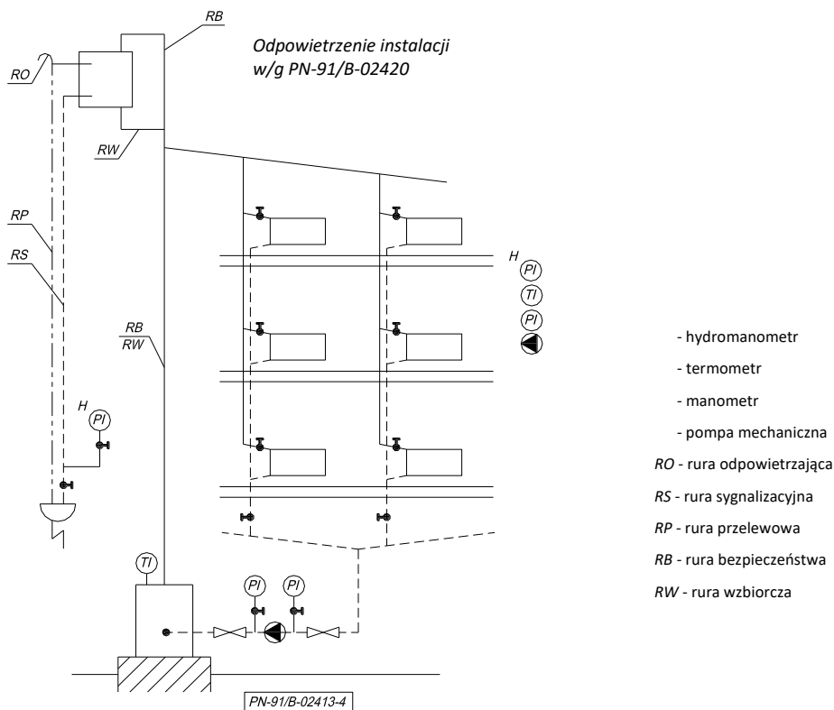
Rys. 2. Przykładowy schemat zabezpieczenia instalacji ogrzewania wodnego, wyposażonej w jeden kocioł, rozdział górny, pompa zamontowana na powrocie.
