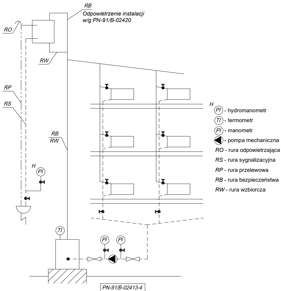
Rys. 4d. Przykładowy schemat zabezpieczenia instalacji ogrzewania wodnego, wyposażonej w jeden kocioł, rozdzielacz górny, pompa zamontowana na powrocie
