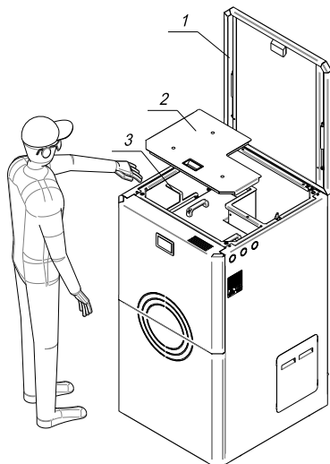
Rys. 8. Schemat mechanicznego czyszczenia wymiennika kotła PERŁA
