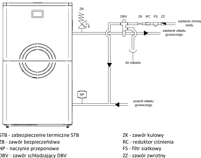
Rys. 4f. Przykładowy schemat zabezpieczenia instalacji ogrzewania wodnego, wg normy PN-EN 12828
