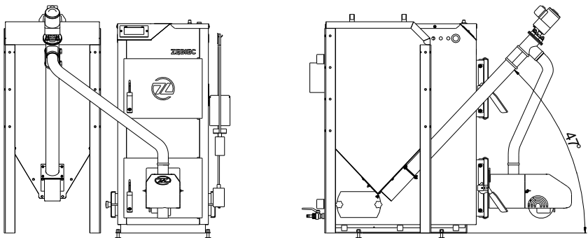
Rys. 4. Sposób ustawienia kosza i zewnętrznego podajnika paliwa.
