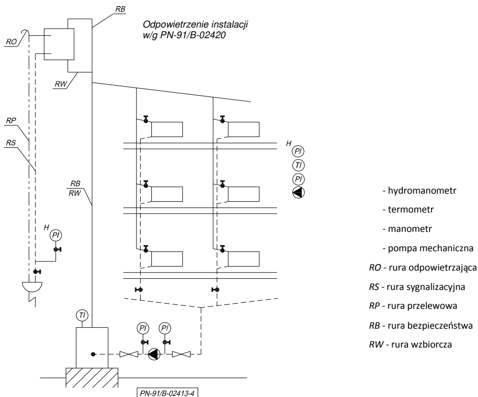
Rysunek 3a. Przykładowy schemat zabezpieczenia instalacji ogrzewania wodnego, wyposażonej w jeden kotłó, rozdzielacz górny, pompa zamontowana na powrocie.
