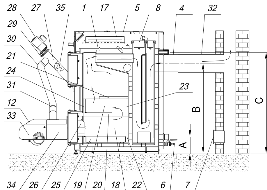
Rys. 3. Schemat oraz typowe podłączenie kotła AGAT.
