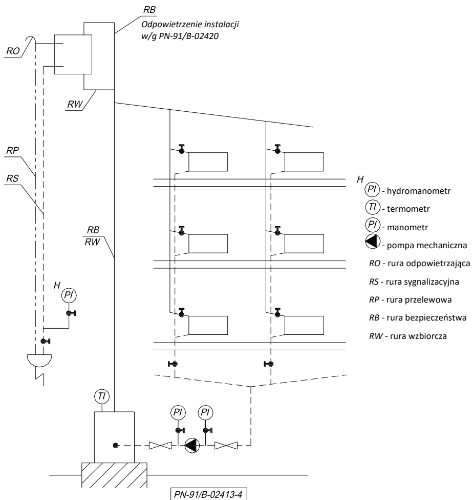
Rys. 2. Przykładowy schemat zabezpieczenia instalacji ogrzewania wodnego, wyposażonej w jeden kotłó, rozdział górny, pompa zamontowana na powrocie.
