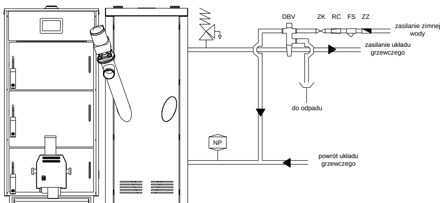
Rys. 7. Przykładowy schemat zabezpieczenia instalacji ogrzewania wodnego, wg normy PN-EN 12828
