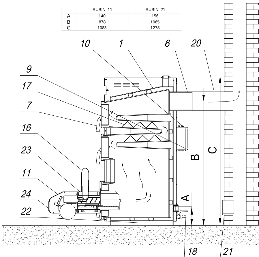
Rysunek 8. Schemat oraz typowe podłączenie kotła RUBIN
