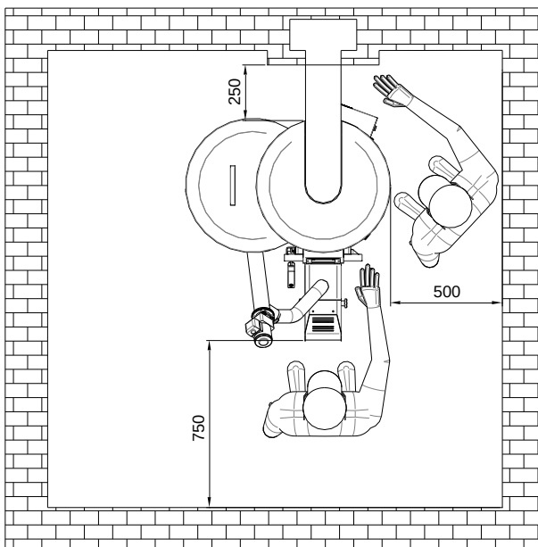
Rysunek 3. Minimalne odległości kotła DIAMENT od ścian kotłowni
