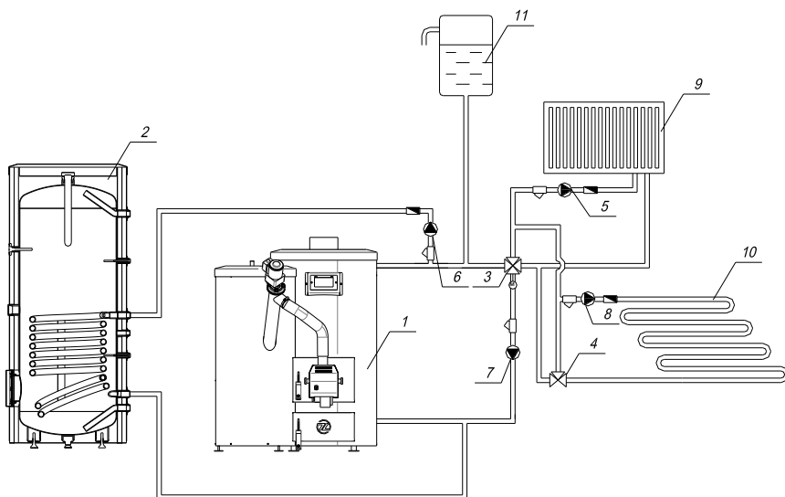
Rys. 6. Uproszczony schemat instalacji grzewczej systemu otwartego
